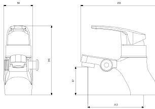
BL3-3601 원홀세면샤워기
