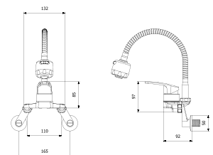
BL3-8001 자바라
