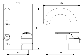
BL2-4604 거위목세면샤워기
