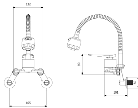
BQ3-8001 자바라
