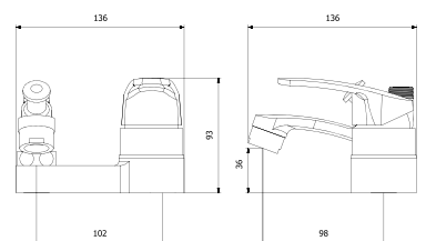
BL3-4601 세면샤워기
