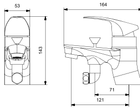
BS3-3601 원홀세면샤워기
