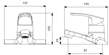
BL3-4001 세면기
