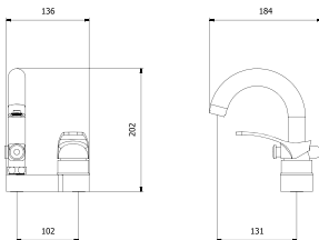
BS2-1-4604 거위목세면샤워기
