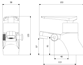
BQ3-3601 원홀세면샤워기
