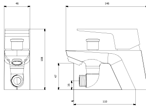
Bβ-3601 원홀세면샤워기
