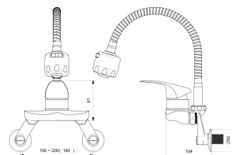
BS3-8001 자바라
