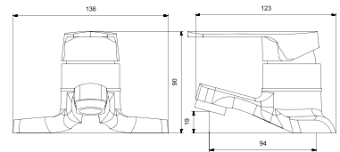
BL2-4001 세면기
