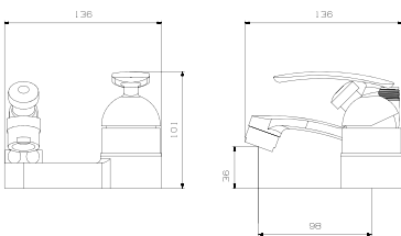
BL1-4601 세면샤워기
