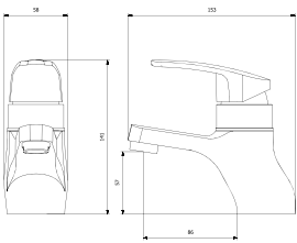
BL3-3001 원홀세면기
