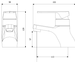
BL2-3001 원홀세면기
