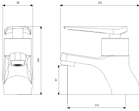
BQ3-3001 원홀세면기
