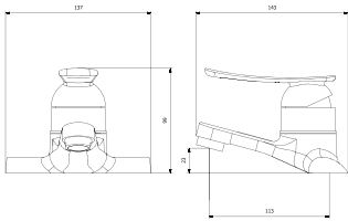
BL4-4001 세면기
