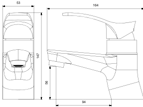
BS2-1-3001 원홀세면기
