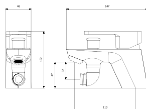
Bβ2-3601 원홀세면샤워기
