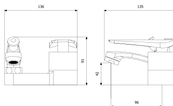
BQ3-4601 세면샤워기
