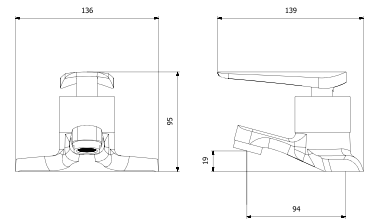
BQ3-4001 세면기
