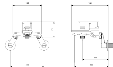
Bβ2-6001 샤워기
