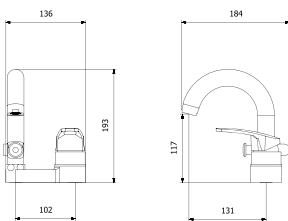
BL3-4604 거위목세면샤워기
