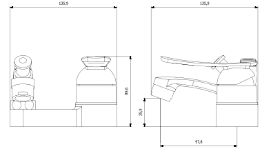
BL4-4601 세면샤워기
