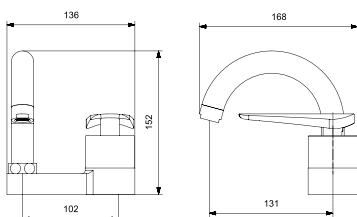
BQ3-4004 거위목세면기
