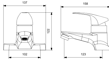
BS3-4001 세면기
