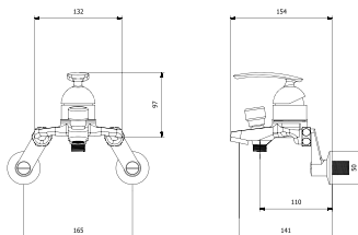
BL1-6001 샤워기
