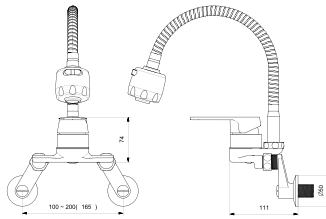
BL2-8001 자바라
