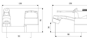
BL2-4601 세면샤워기
