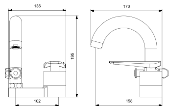
BQ3-4604 거위목세면샤워기
