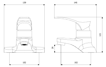
BS2-1-4001 세면기
