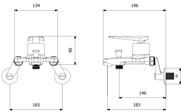
BQ3-6001 샤워기
