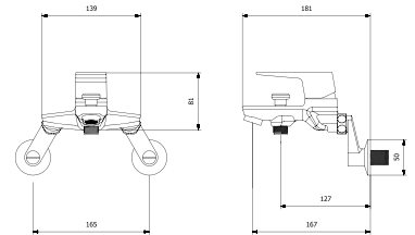
Bβ-6001 샤워기
