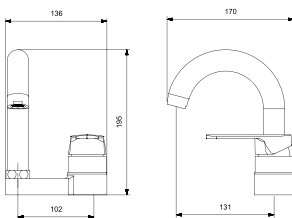
BL2-4004 거위목세면기
