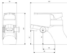
BL2-3601 원홀세면샤워기
