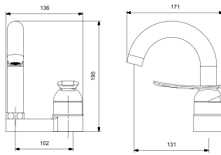
BL4-4004 거위목세면기
